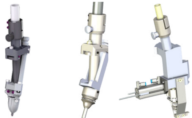
2-Backen 110° Mundstück mit Ambos und Schwenkarm
