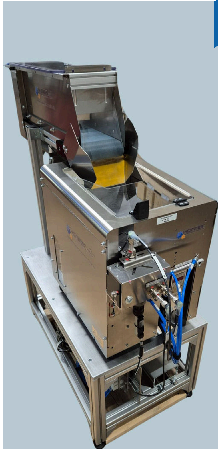
Zuführstation mit Füllbunker
