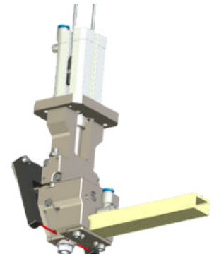
Mundstück für eine Mutter Setzeinheit
